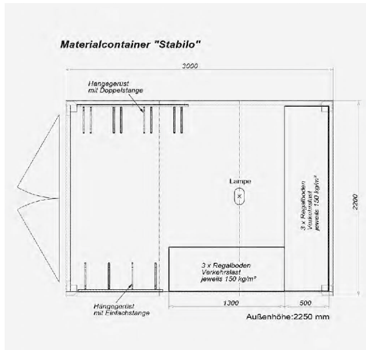
Beispielhafte Ausstattung und Raumaufteilung des Materialcontainers „STABILO“.
